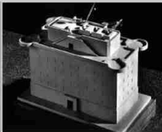
G-Turm I Berlin-Tiergarten : L-Turm I Berlin-Tiergarten Bauzeit: Oktober 1940 - April 1941
